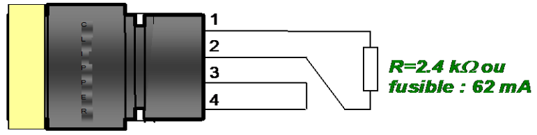
Connecteur mâle
